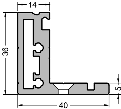
Profil ist unten alle 375 mm vorgebohrt Profile is pre-drilled at the bottom every 375 mm
