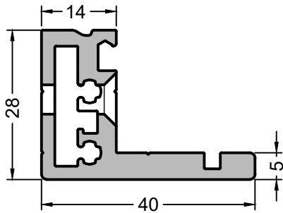
Profil ist seitlich alle 75 mm vorgebohrt Profile is pre-drilled at the side every 75 mm
