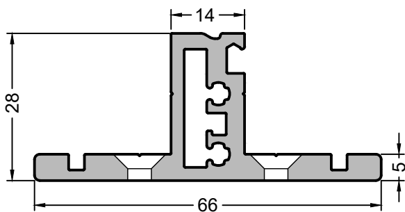
Profil ist unten alle 75 mm vorgebohrt Profile is pre-drilled at the bottom every 75 mm
