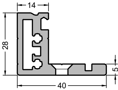
Profil ist unten alle 75 mm vorgebohrt Profile is pre-drilled at the bottom every 75 mm
